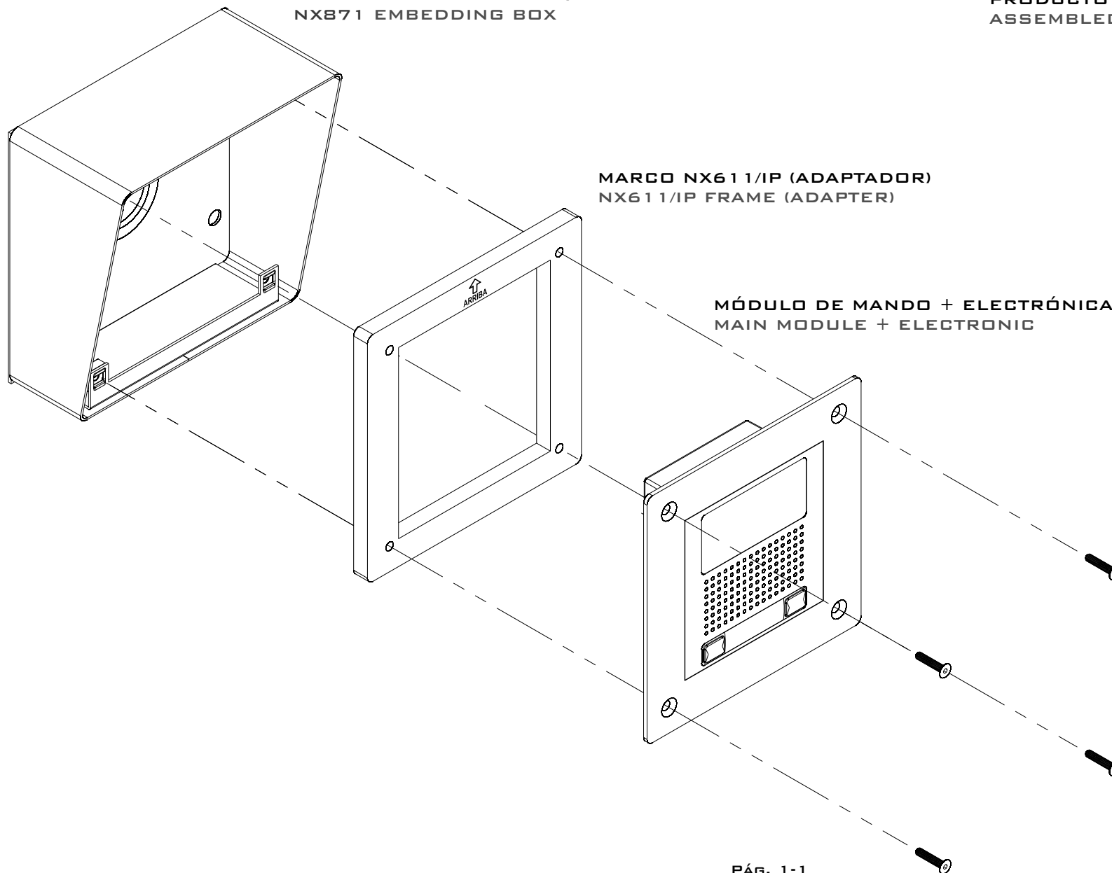
CAJA DE EMPOTRAR NX871 NX871 EMBEDDING BOX
