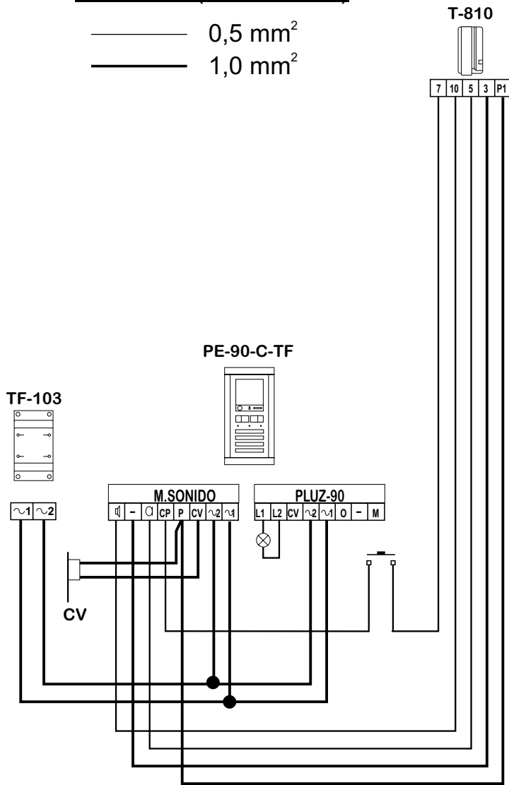
Llamada por zumbador / Buzzer Calling.
