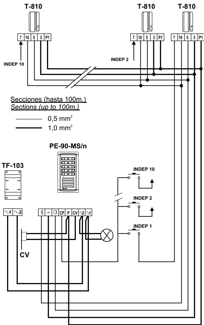
Llamada por zumbador / Buzzer Calling.
